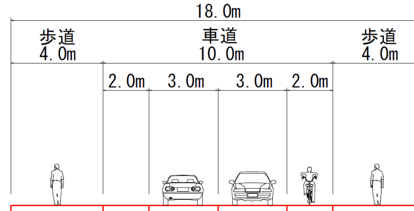
標準断面図
