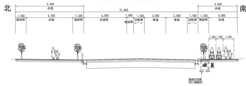
計画標準断面図
