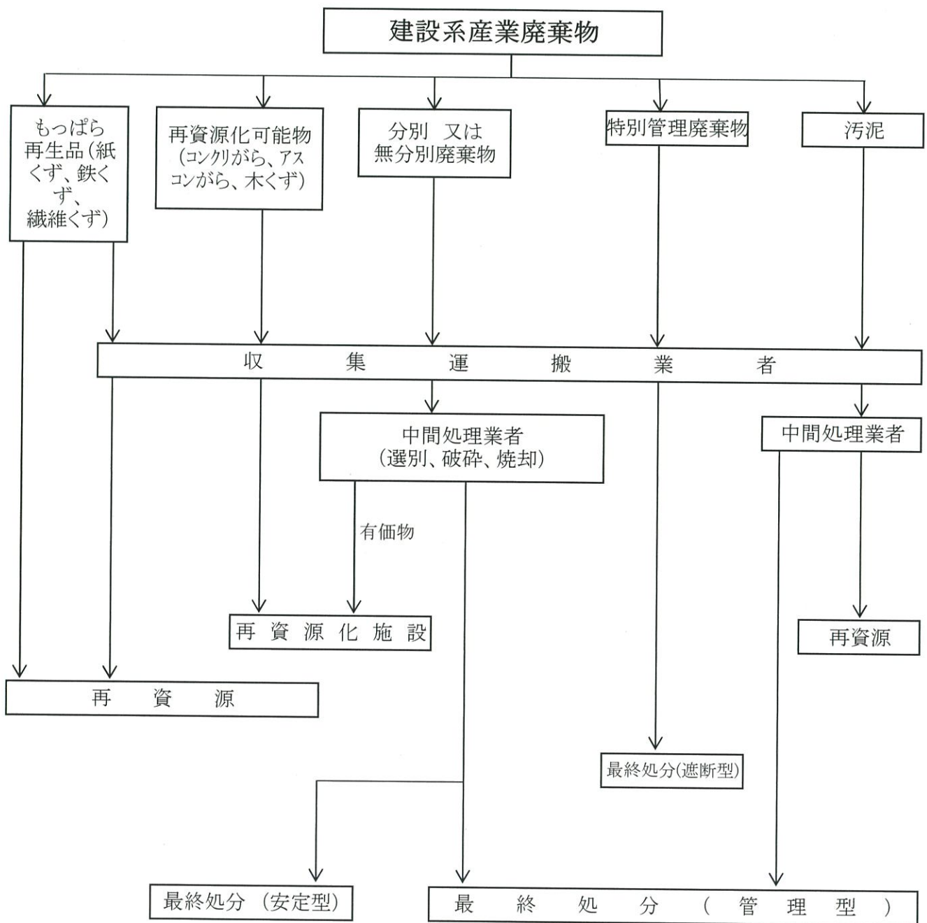
(第1面)4産業廃棄物の一連の処理の工程
