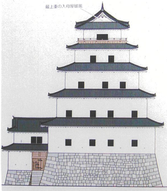
丹波亀山城 最上階以外の破風のない天守。 5重5階 左南面 右西面（初期層塔型天守）（図は「天守のすべて①学研」より）
