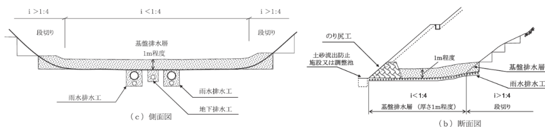
図 2.42 基盤排水層の設置例
