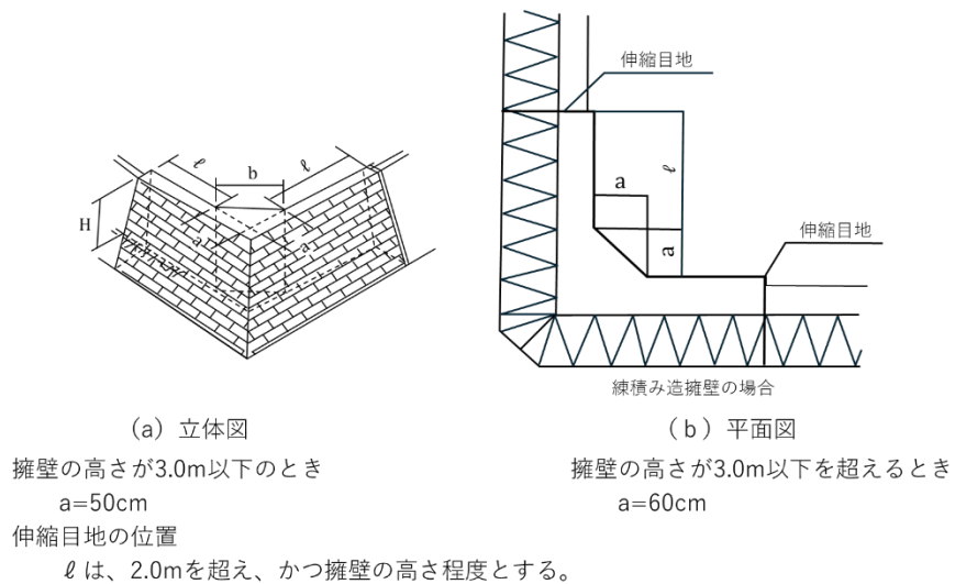
図 2.33 隅角部の補強方法及び伸縮継目の位置
