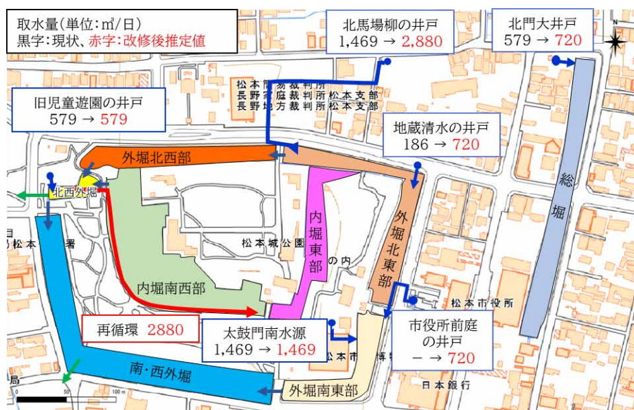
松本城堀における再循環
