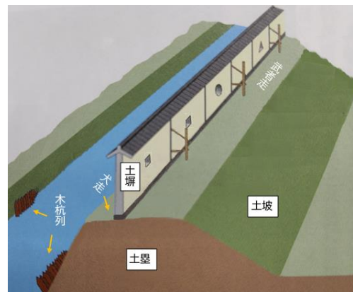
土塁と土堀のイラスト図
