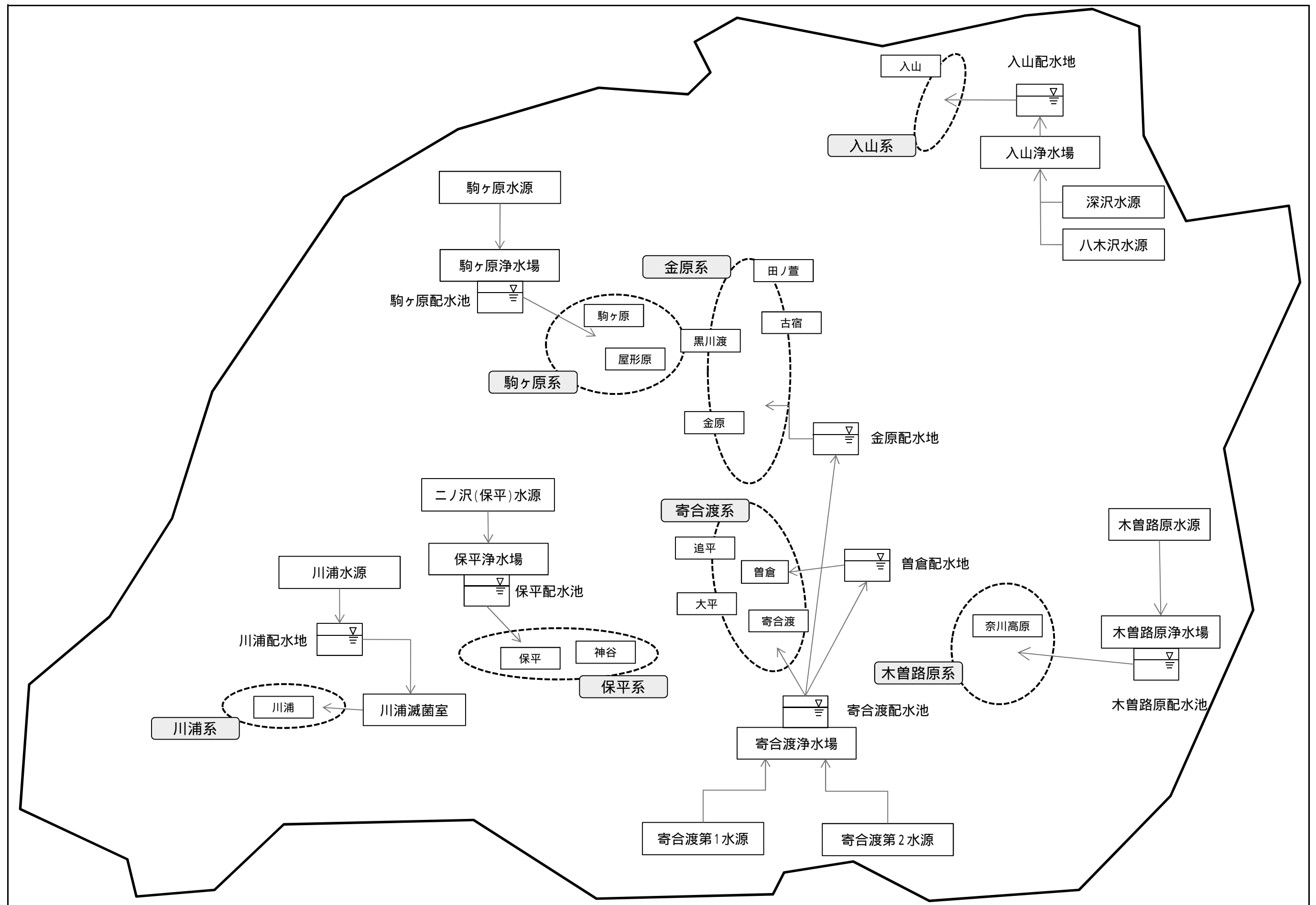
(3 - 3) 梓川地区水道事業(奈川)配水系統概要図
