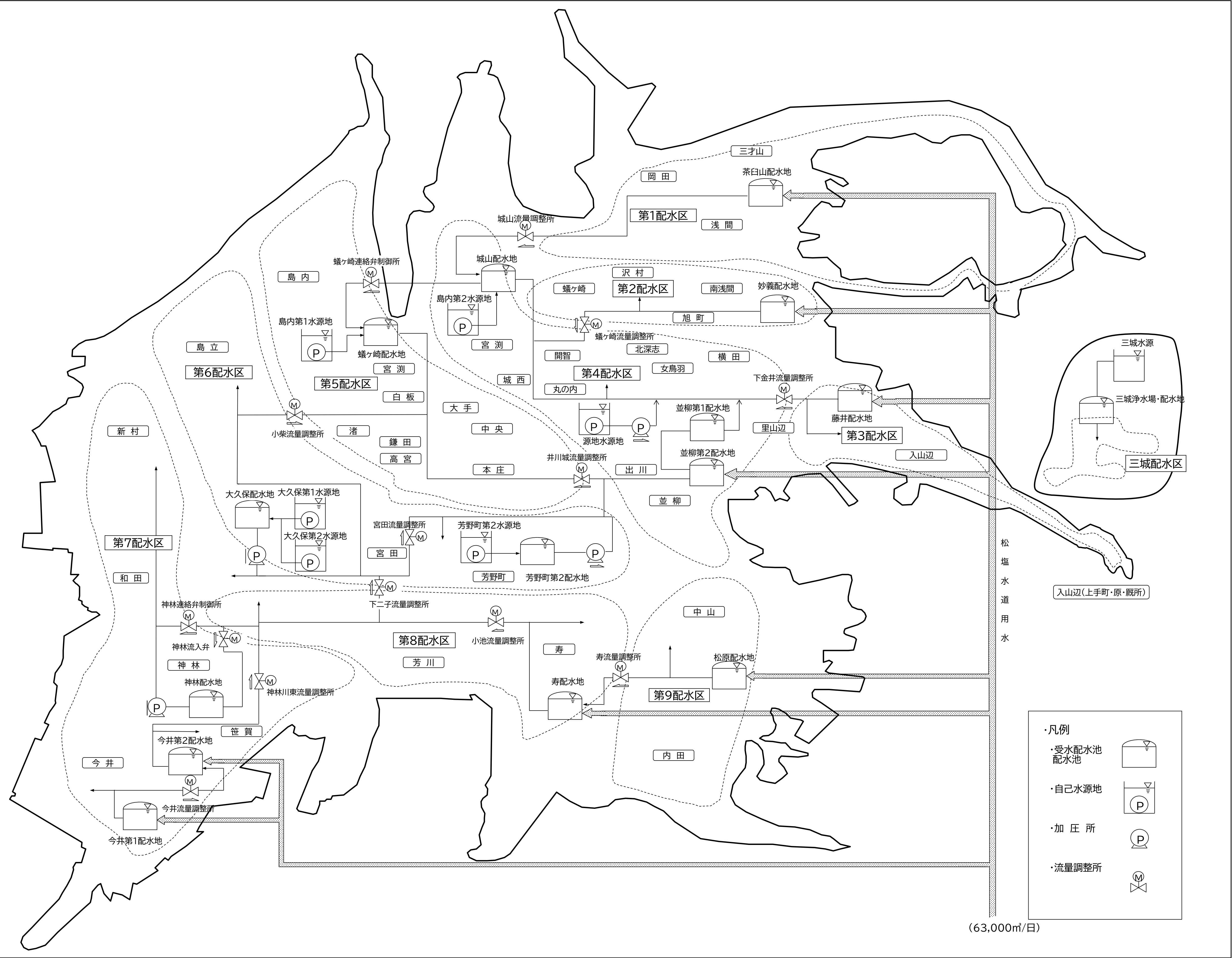
(1) 松本地区水道事業配水系統概要図
