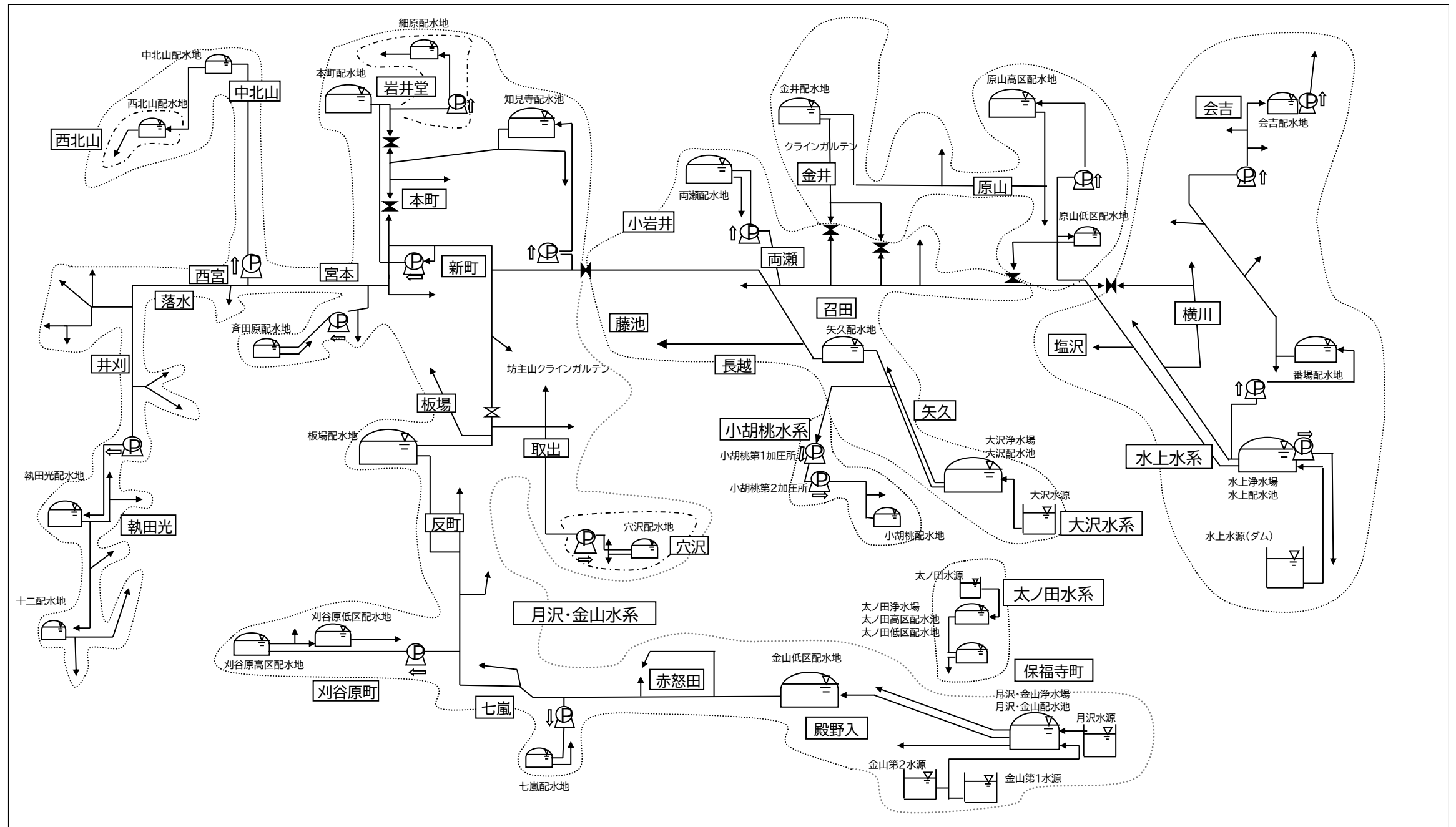
(2)四賀地区水道事業配水系統概要図
