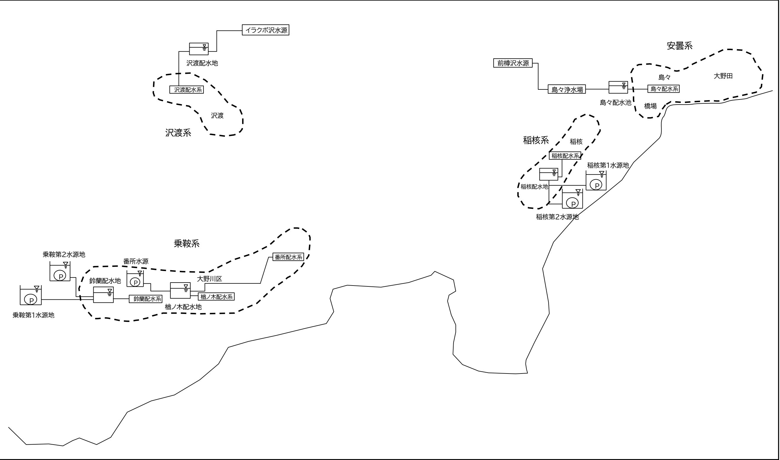
(3-2)梓川地区水道事業(安曇)配水系統概要図
