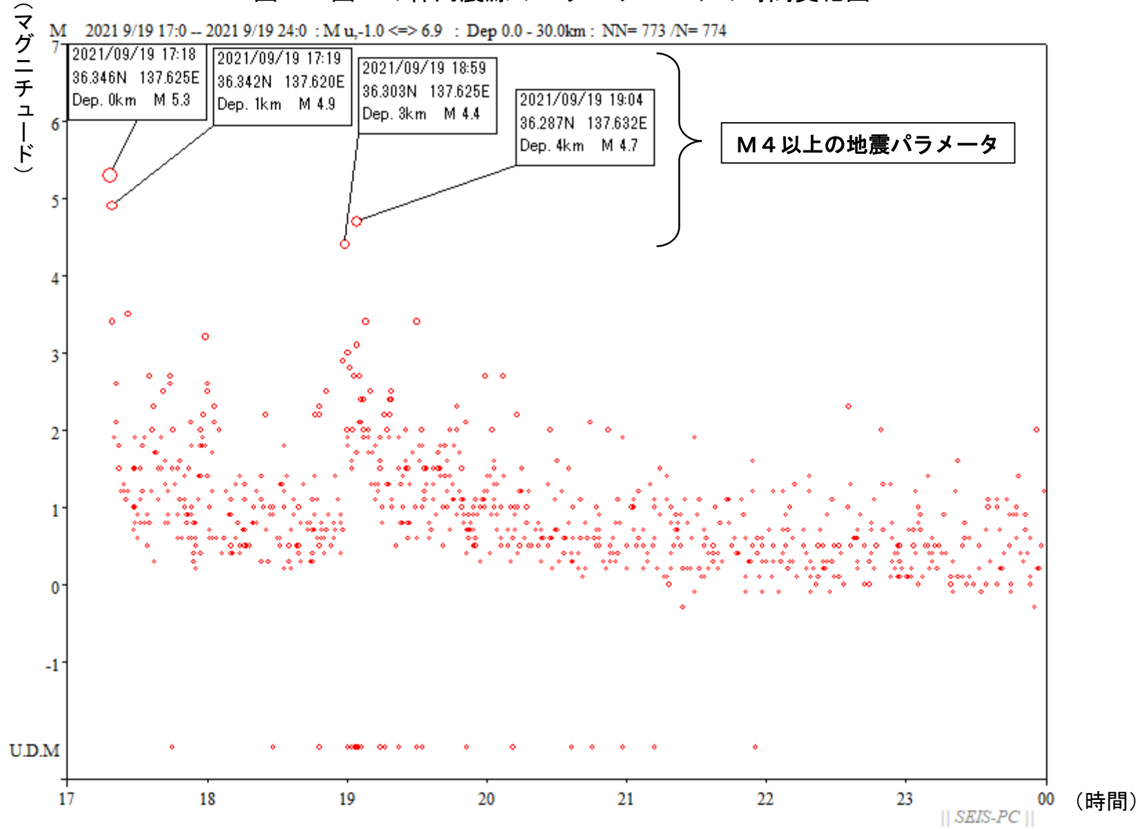
図3：図1の枠内震源のマグニチュードの時間変化図
