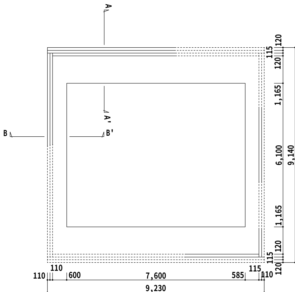
平面図
