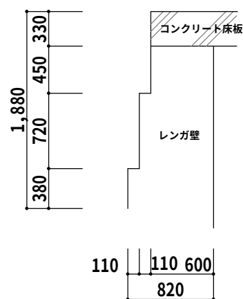
B-B'
