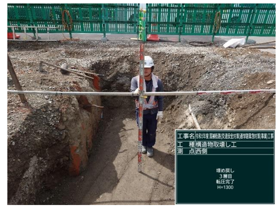
西壁面 取り壊し状況
