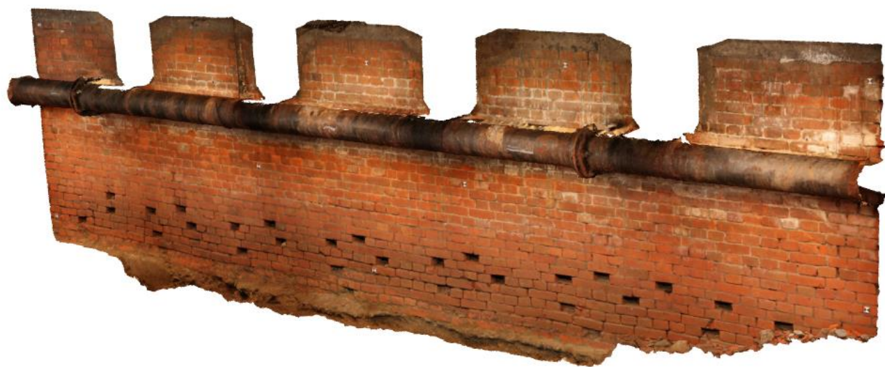
南壁
